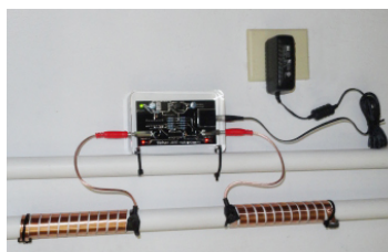
Bild 4: Grundsätzliche Anordnung zur physikalischen Wasserbehandlung
